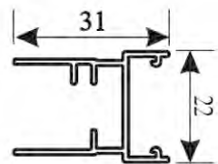
05 PROFIL BOCZNY Z SIATKĄ
