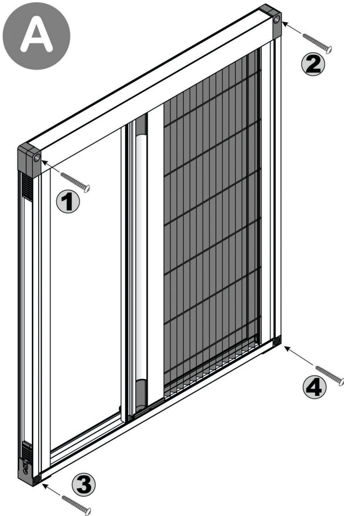
PUNKTY MOCOWANIA
